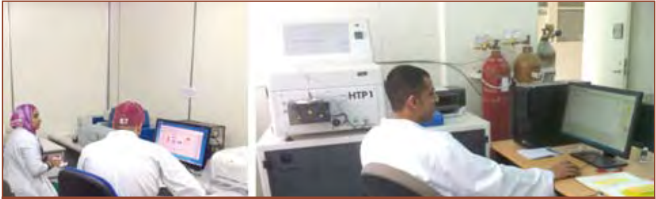
صور مجمعة أخذت لتبين عدداً من أجهزة الاختبارات المستخدمة في تعيين خواص حبيبات هيدريد المغنيسيوم النانوية ومتراكباتها وذلك في مختبرات تكنولوجيا النانو التابعة لمركز أبحاث الطاقة والبناء بمعهد الكويت للأبحاث العلمية
