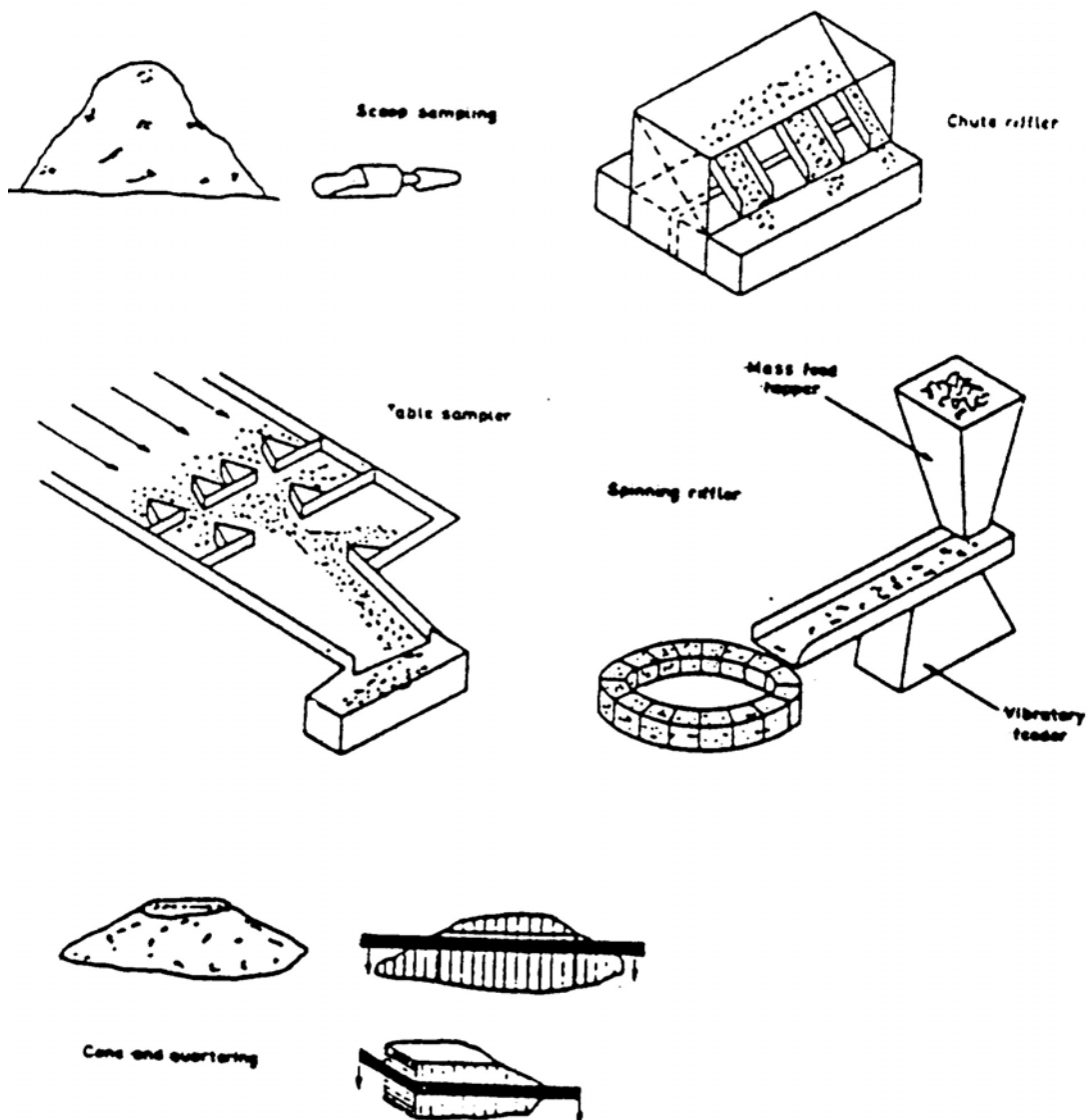
الشكل (٢ - ٣): طرق تجزئة العينة للحصول على العينة النهائية للتحليل
