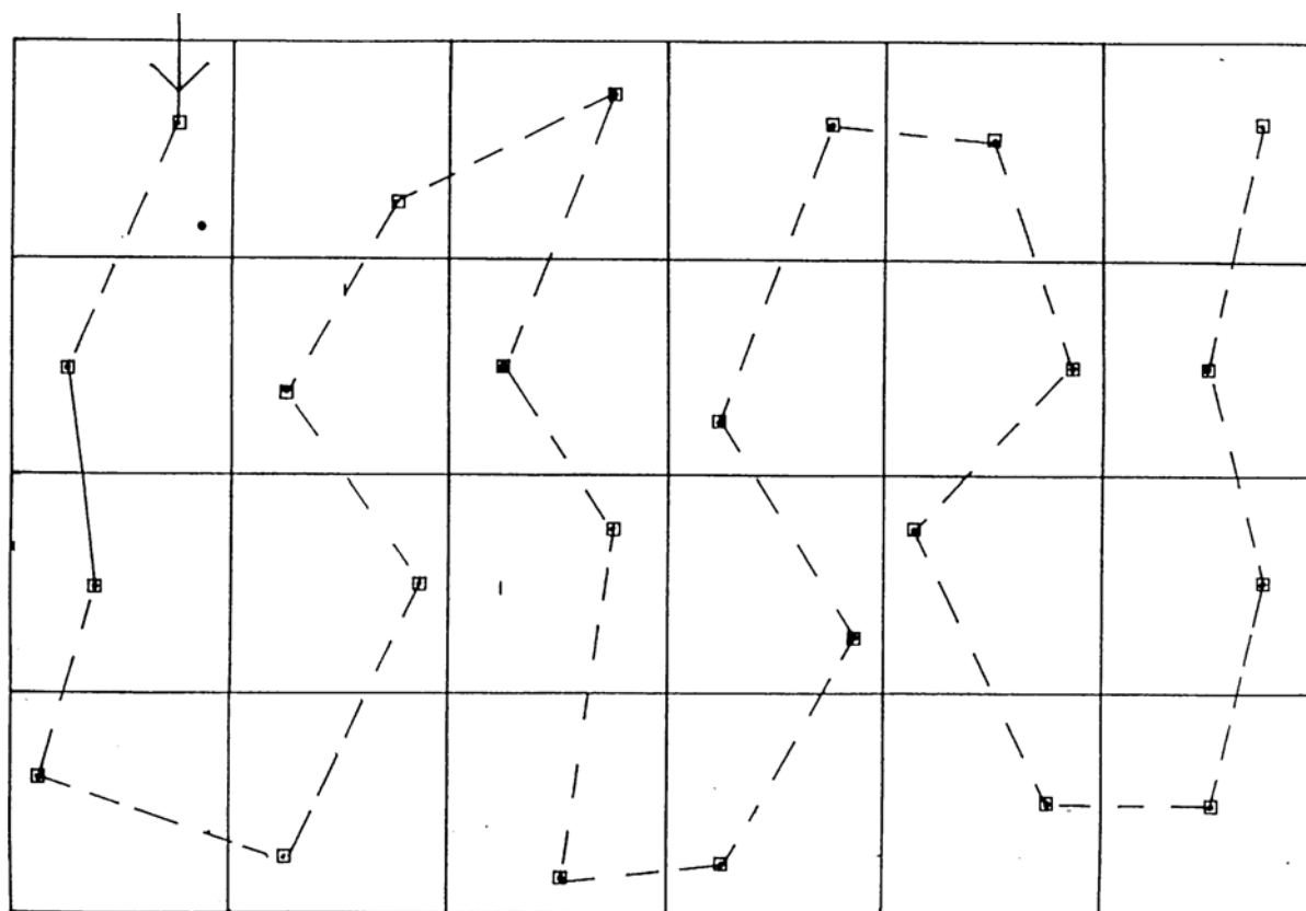
الشكل (٢ - ١): طريقة أخذ عينات التربة على شكل حرف W
