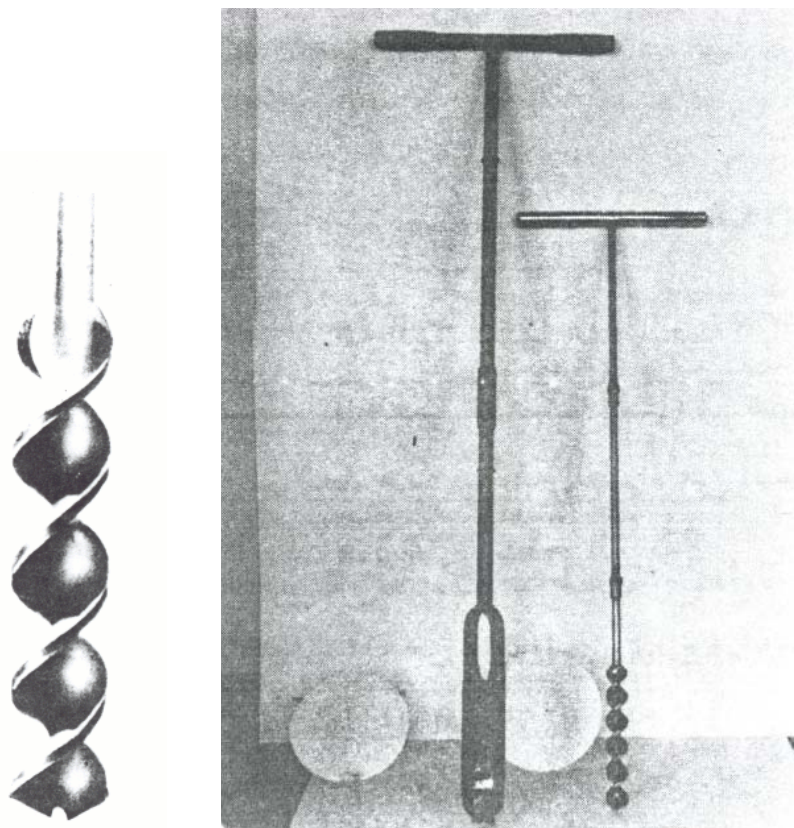
الشكل (٢ - ٢): البريمة
