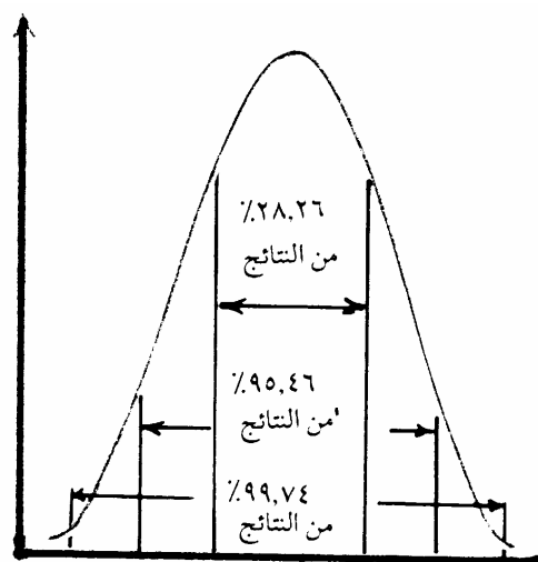
الشكل (١): شكل المنحنى الطبيعي
