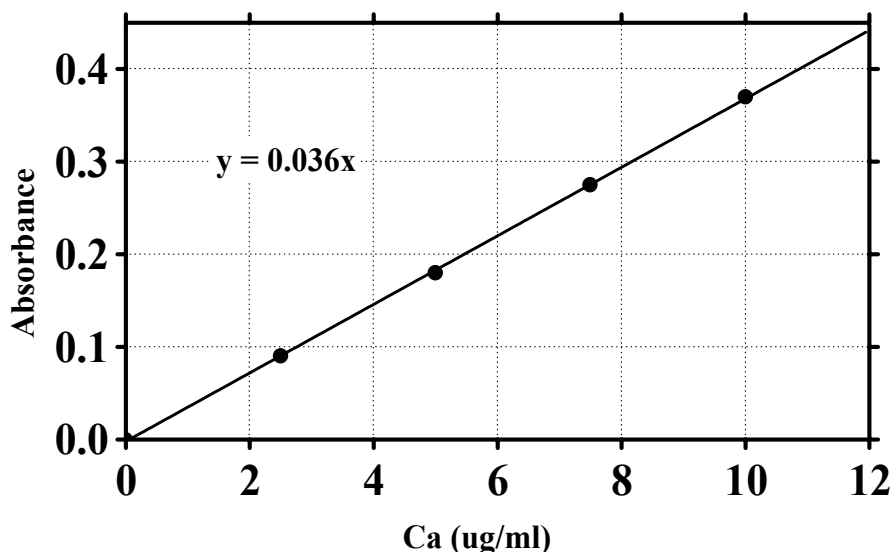
الشكل (٤ - ٣): منحنى التدرج القياسي للكالسيوم
